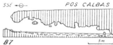
Fig. 35. Doorsnede in ZZO–NNW richting van de grot van Pos Calbas (B 7), op de plantage Lima, Bonaire. — De kalksteen is gearceerd, het water horizontaal gestreept.
